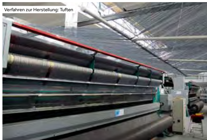
Aufwickeln der getufteten Oberfläche
